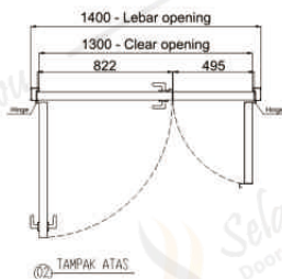
02 TAMPAK ATAS
