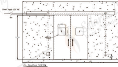
Double Door
