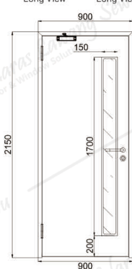
01 TAMPAK DEPAN
