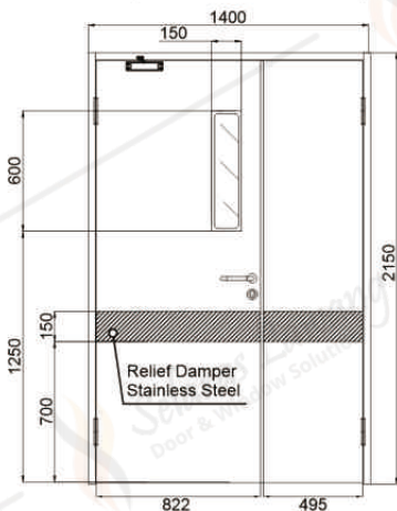
01 TAMPAK DEPAN
