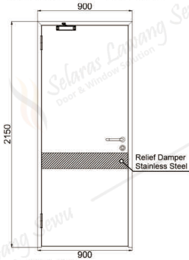
01 TAMPAK DEPAN
