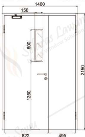
01 TAMPAK DEPAN
