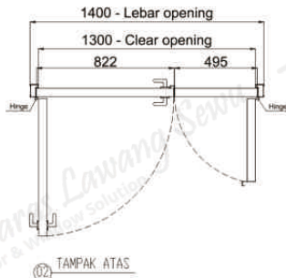
02 TAMPAK ATAS
