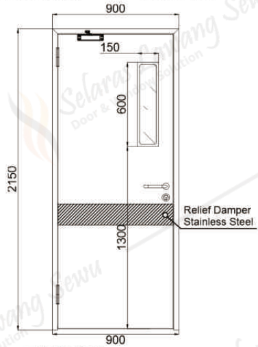
01 TAMPAK DEPAN
