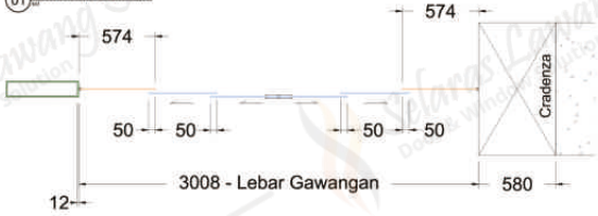
02 TAMPAK ATAS
