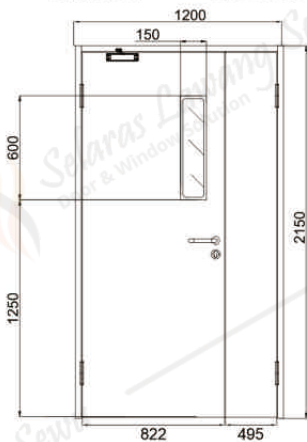
01 TAMPAK DEPAN
