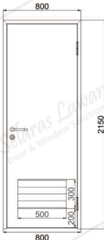
01 TAMPAK DEPAN
