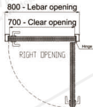
02 TAMPAK ATAS
